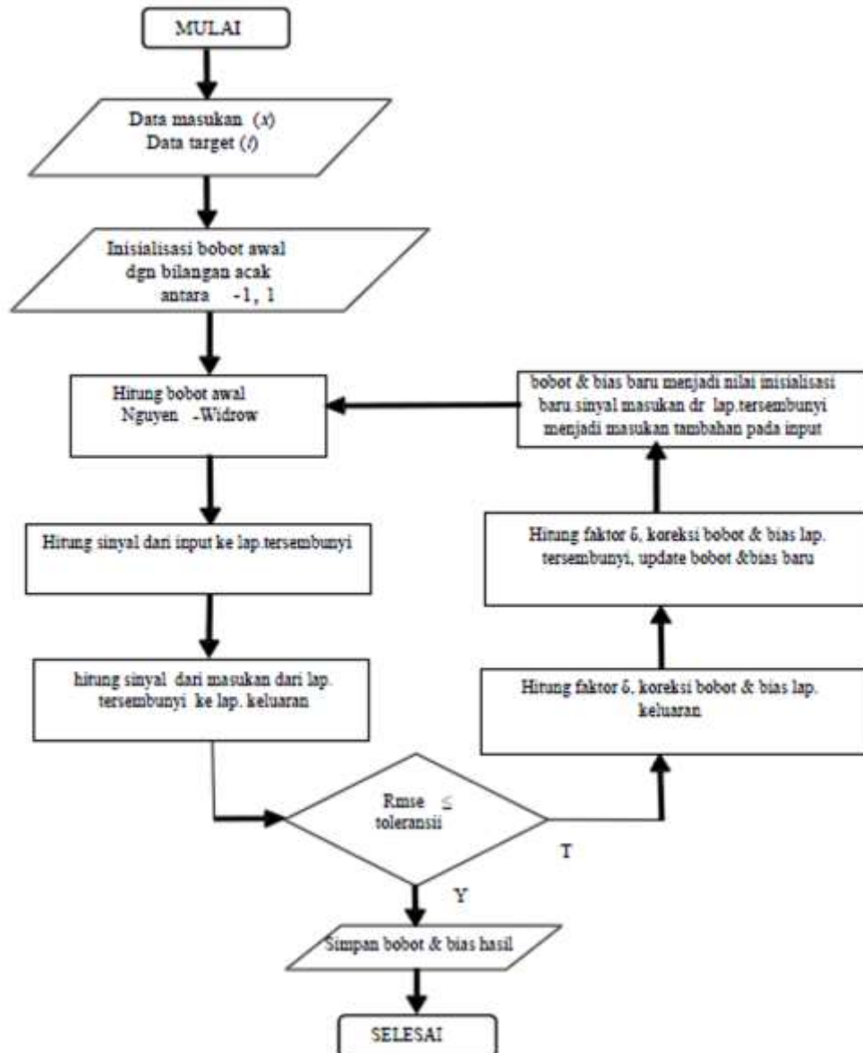
Gambar 4. Flowchart proses pelatihan jaringan
