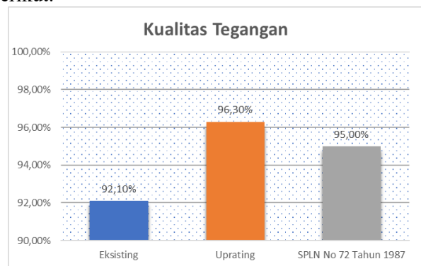
Gambar 7. Grafik Perbandingan Kualitas Tegangan Setelah Uprating
