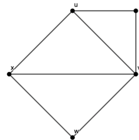
Gambar 1. Graf G
