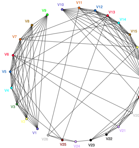
Gambar 5. Pewarnaan Graf
