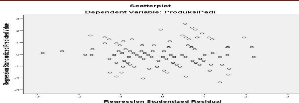
Gambar 3. Uji Heteroskedastisitas
