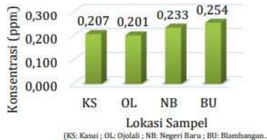
Gambar 1. Kandungan Logam Pb dalam Air Sungai Way Umpu
