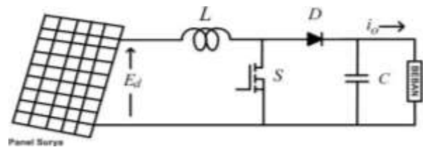
Gambar 6. Rangkaian beban DC chopper boost
