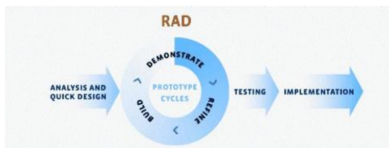
Gambar 1. Metode RAD
