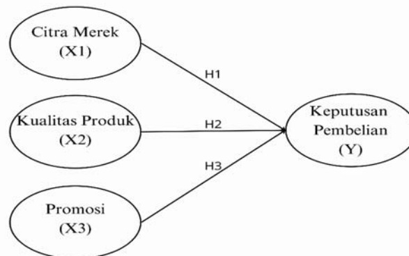
Gambar 3. Kerangka Konseptual.
