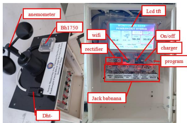
Gambar 11: Tampilan Alat Dari Atas dan Dalam Box
