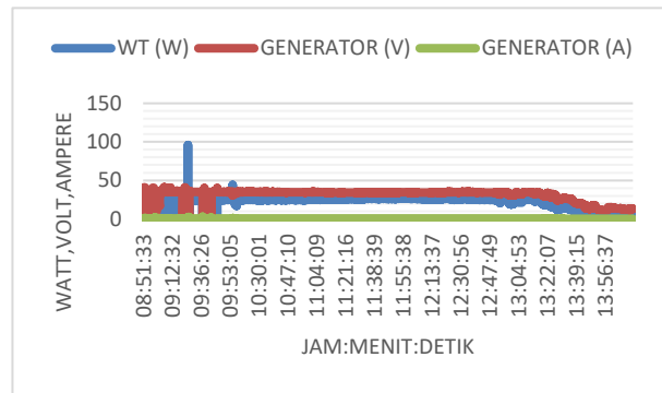
Gambar 15: Data Pengujian Pada Tanggal 26 Oktober 2023
