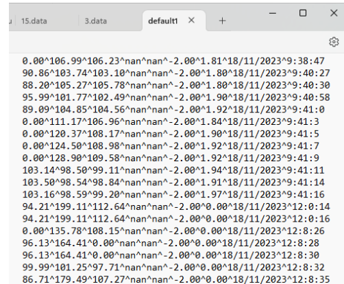
Gambar 10: Hasil Penulisan DataRecord
