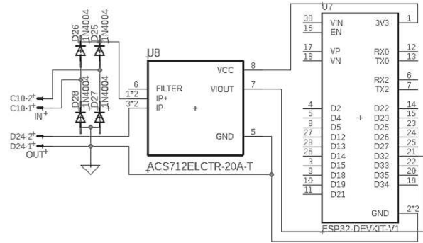
Gambar 3 Merupakan Rangkaian Sensor Arus ACS712 5amp
