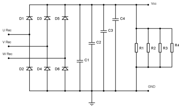
Gambar 5 Merupakan Rangkain Rectivier 3 Phasa
