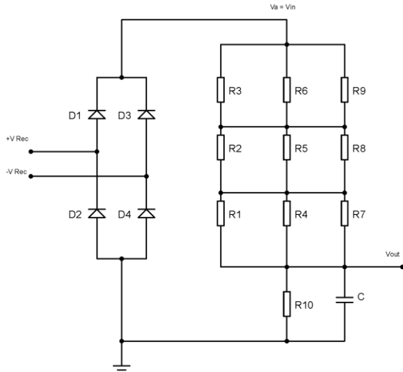
Gambar 2 Merupakan Gambar Rangkaian Sensor Tegangan Turbin angin Generator
