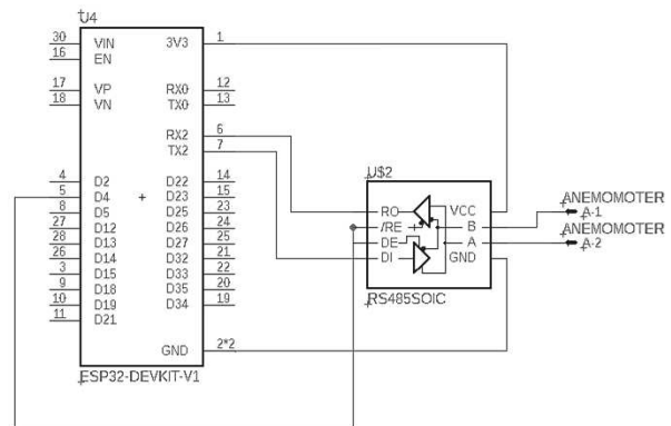
Gambar 4 Merupakan Rangkaian Sensor Anemometer RS-FSJT-N01
