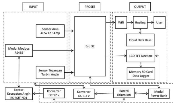
Gambar 1 Merupakan diagram blok pada sistem penelitian yang meliputi input, proses dan output
