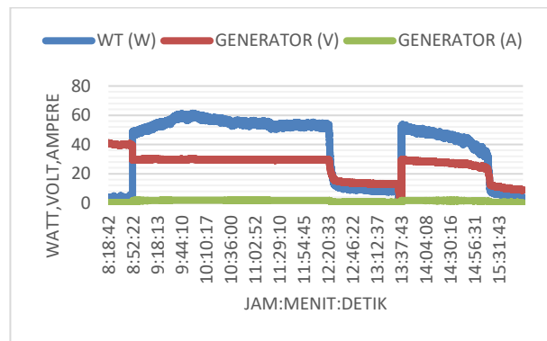
Gambar 16: Data Pengujian Pada Tanggal 27 Oktober 2023
