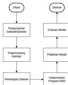
Gambar 1. Flow Metode yang diusulkan
