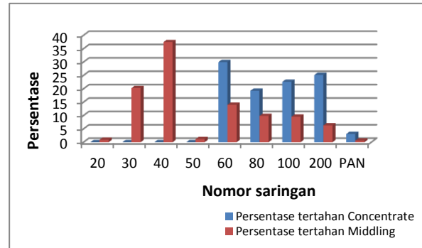
Gambar 4. Grafik perbandingan material tertahan pada setiap nomor saringan
