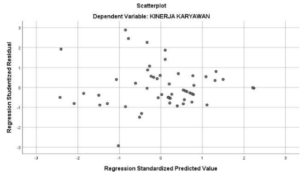
Gambar 2 Uji Heterokedastisitas
