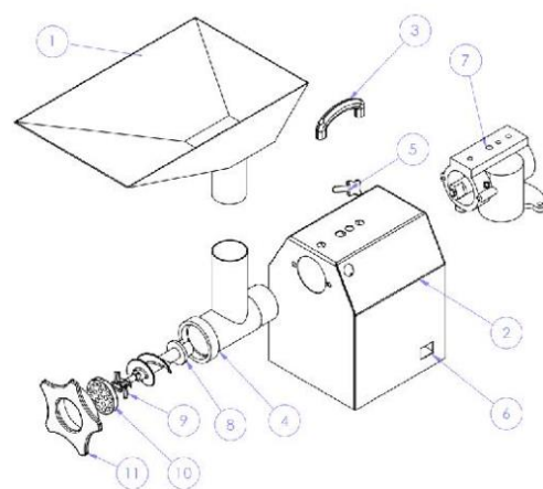
Gambar 7. Komponen Mesin Pengaduk
