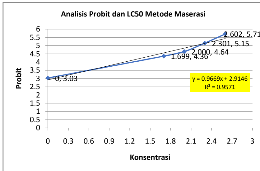
Gambar 1. Grafik Regresi Linier Konsentrasi Ekstrak Etanol Daun Kratom Metode Maserasi.
