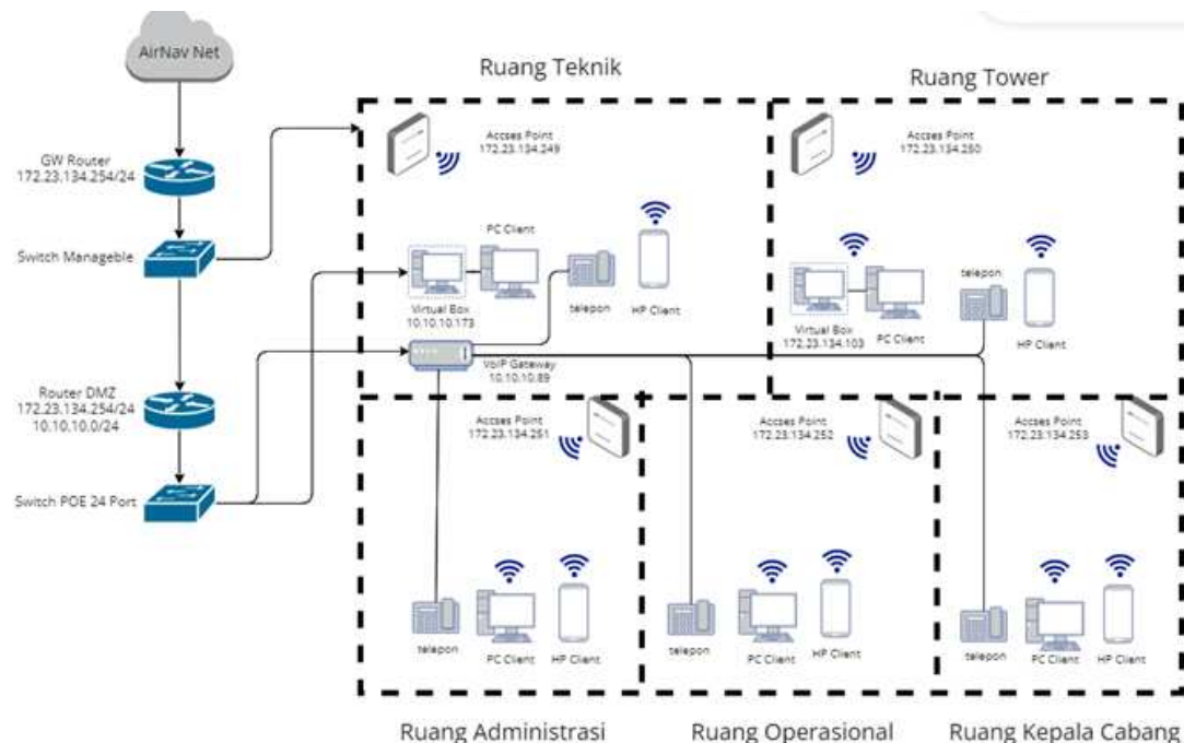
Gambar 1. Topologi rancangan VoIP server
