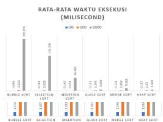
Gambar 15. Rata-rata Waktu Eksekusi pada 6 algoritma sorting
