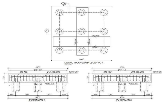
Gambar 3 Detail Pekerjaan Pile Cap dan Pondasi Spun Pile Sumber : Data proyek pembangunan gardu induk perawang, 2019
