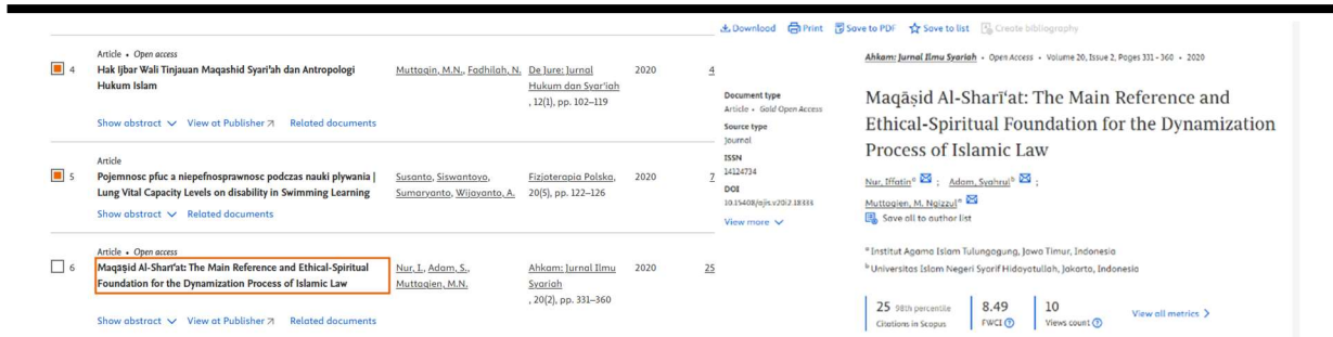
Gambar 3. Filterisasi dokumen
