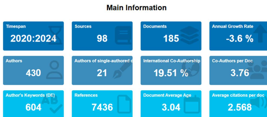
Gambar 5. Informasi utama
