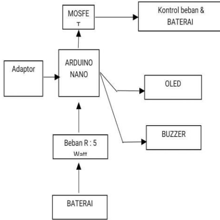
Gambar 3. Blok diagram alat
