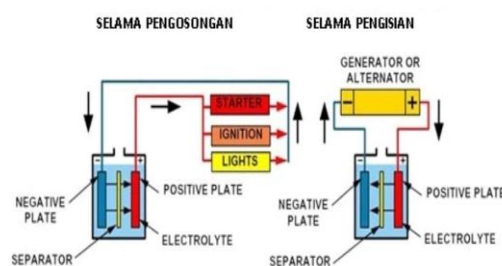
Gambar 1 Proses Pengosongan dan pengisian baterai
