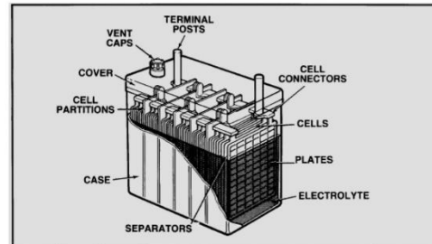
Gambar 2. Kontruksi baterai
