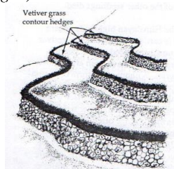
Akar wangi sebagai tanaman pagar penguat teras yang diperkuat tumpukan batu menurut kontur
