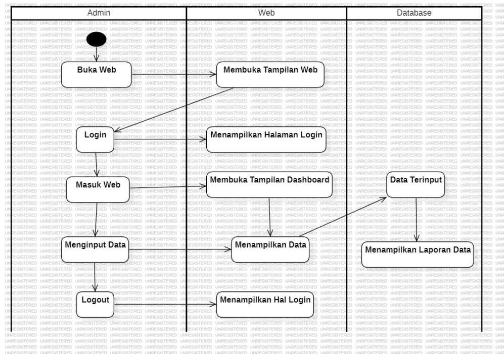
Gambar 5. Diagram Aktivitas
