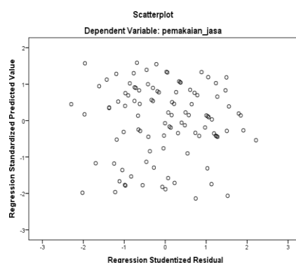
Gambar 2. Uji Heteroskedastisitas
