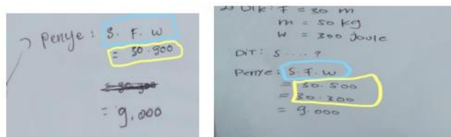
Gambar 2 Kutipan jawaban pada soal nomor 2.
