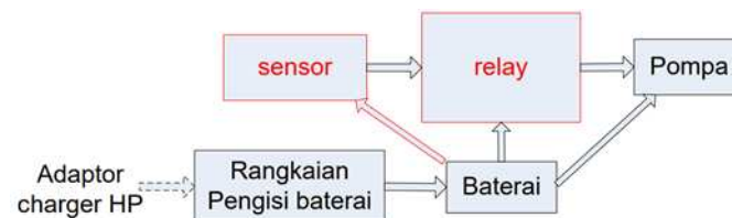
Gambar 8. Bentuk Diagram Sistem Modifikasi
