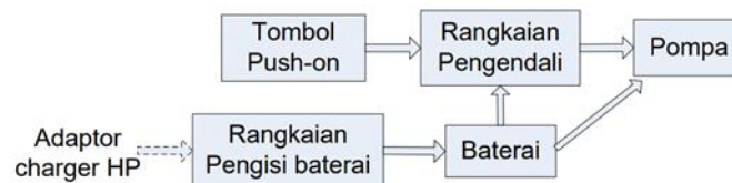
Gambar 7. Diagram Sistem Awal
