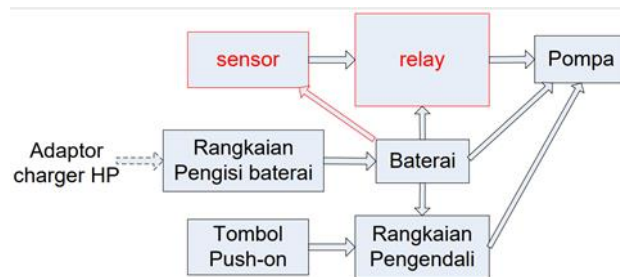
Gambar 9. Bentuk Diagram Keseluruhan
