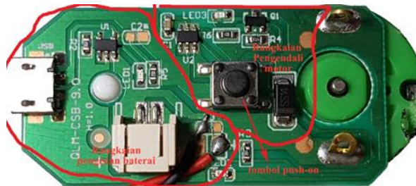
Gambar 6. Bentuk Rangkaian Elektrik Pompa Air Listrik
