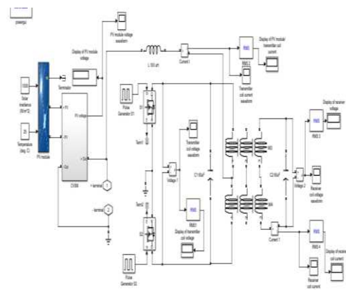
Gambar 4. Model Keseluruhan PVWPT Dengan Magnetik Relay
