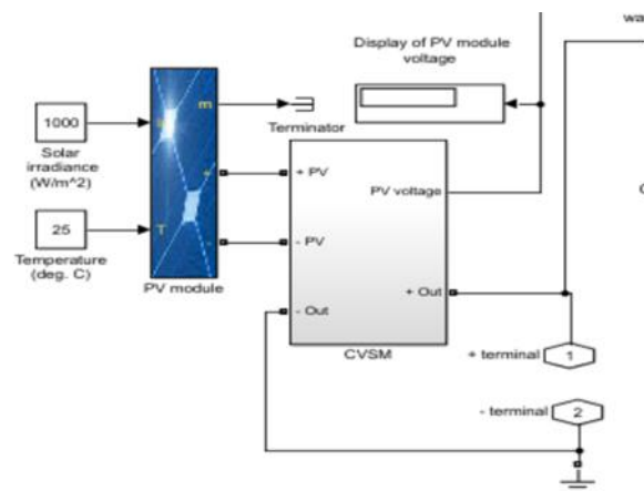
Gambar 1 Modul PV
