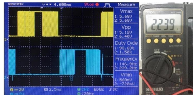
Gambar 5. Gelombang dan tegangan output dari driver MOSFET
