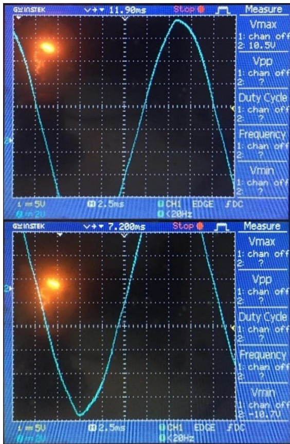
Gambar 12. Gelombang output inverter pure sine wave dengan beban lampu 60 watt
