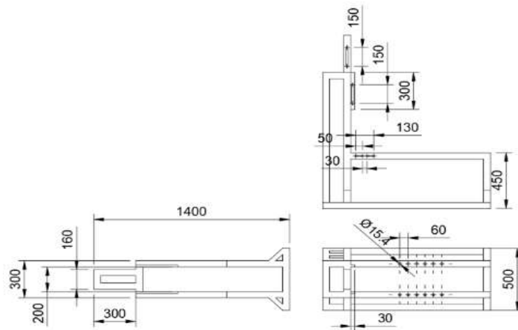
Gambar 6. Desain Kerangka Shock Breaker Traineer Sesudah Dimodifikasi. Hasil penyempurnakaan desain Shock Breaker Traineer sebagaimana Gambar 7.
