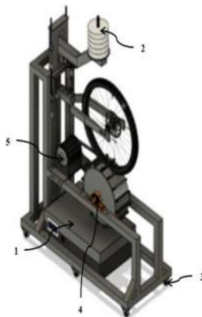
Gambar 6. Desain Kerangka Shock Breaker Traineer Sesudah Dimodifikasi. Hasil penyempurnakaan desain Shock Breaker Traineer sebagaimana Gambar 7.
