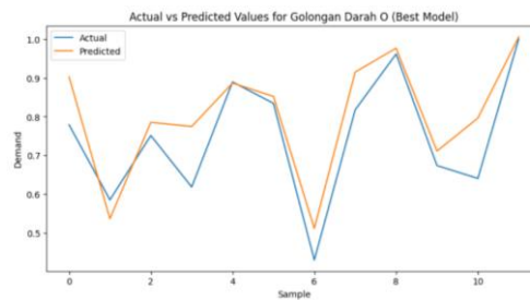
Gambar 4.3 Grafik Aktual vs Prediksi hasil terbaik Golongan Darah O
