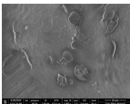
Gambar 8. Hasil SEM Bioplastik dengan berat PP-g-MA 1 gr (perbesaran 2000 X).
