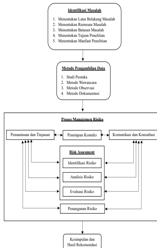
Gambar 1. Metodologi Penelitian
