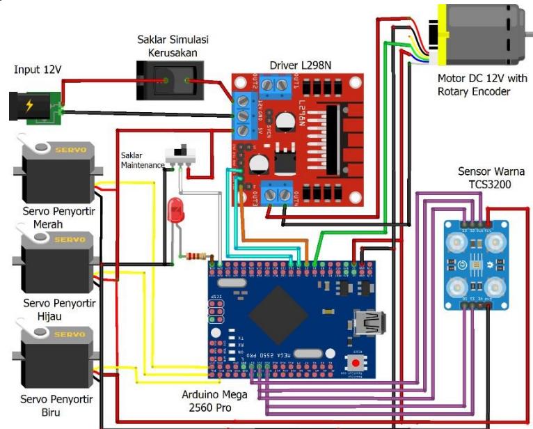
Gambar 6 Rangkaian elektronik
