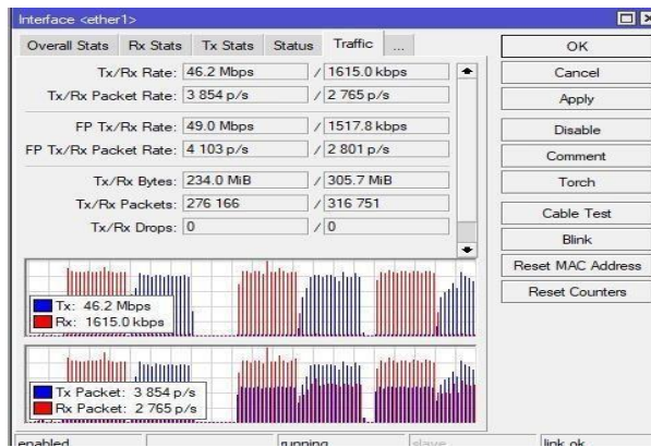
Gambar IV. 25 pengujian jaringan awal
