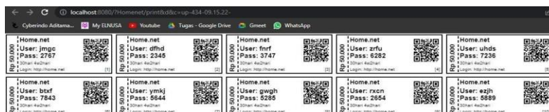
Gambar IV. 22 Generate voucher
