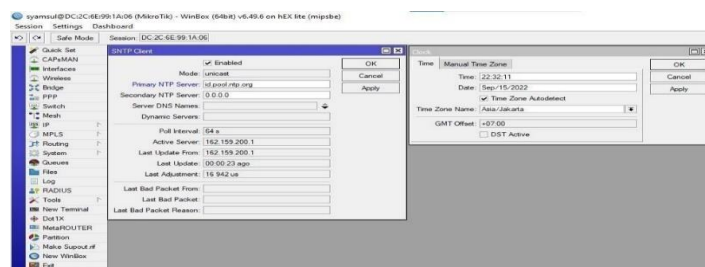
Sumber: Mohammad dzulfikar, 2022 Gambar IV .19 Konfigurasi Waktu
