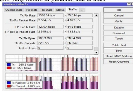
Gambar IV. 26 pengujian jaringan akhir
