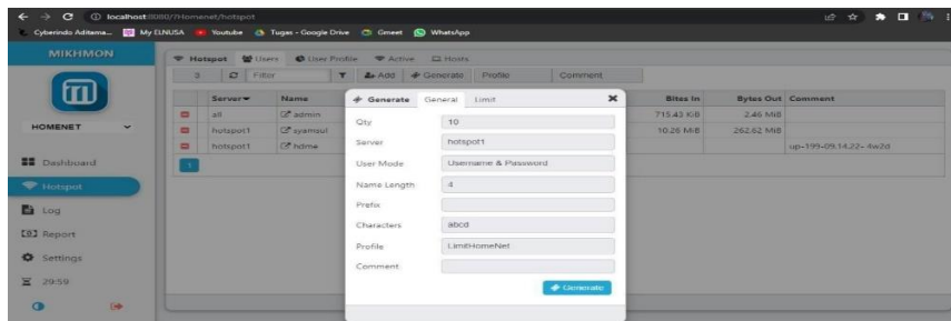
Gambar IV. 22 Generate voucher
