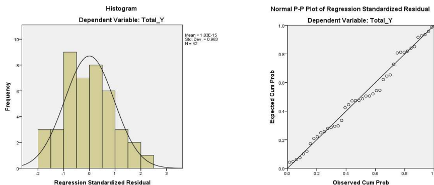
Gambar 2. Uji Normalitas
