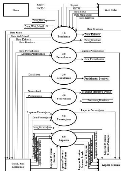
Gambar 3. Diagram Nol Sistem Yang Diusulkan
