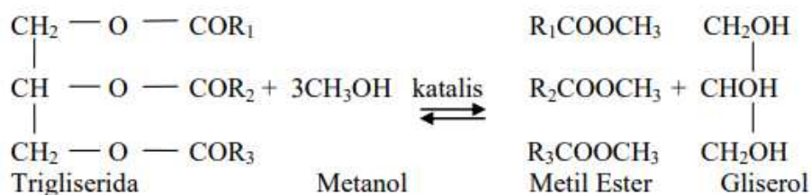
Gambar 4. Pembentuk Gliserol
