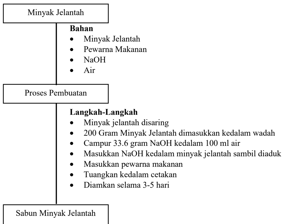
Gambar 5. Diagram Alir Pembuatan Minyak Jelantah
