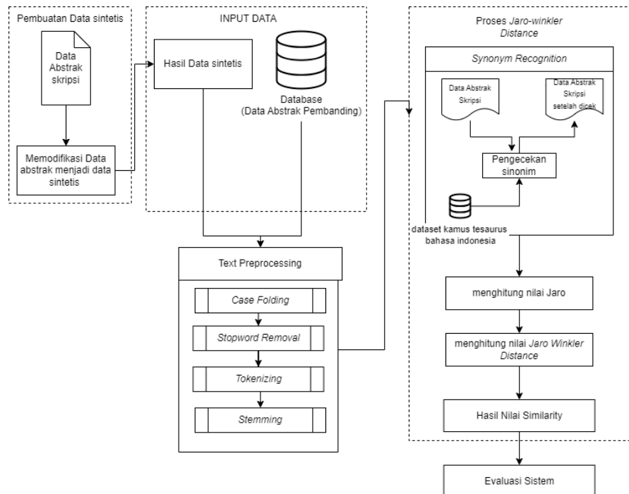
Gambar 2 Arsitektur Sistem
