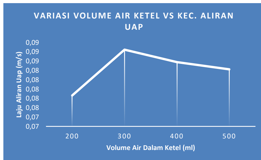
Gambar. 1 Pengaruh Variasi Volume Air terhadap Laju Aliran Uap
