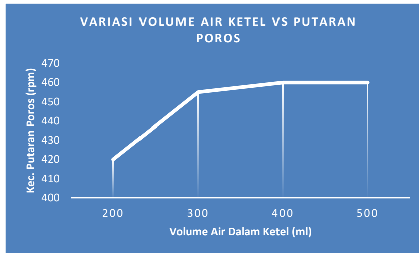
Gambar. 2 Pengaruh Variasi Volume Air terhadap Kecepatan Poros Turbin
