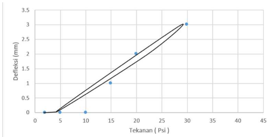
■ Gambar 6 Grafik uji pembebanan rubber damper dengan mesin press hidrolik
