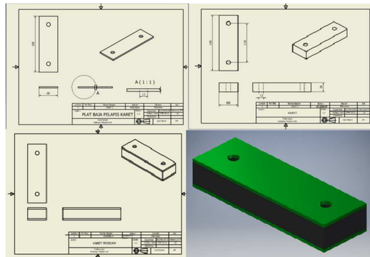
■ Gambar 2 Desain rubber damper lori inspeksi
