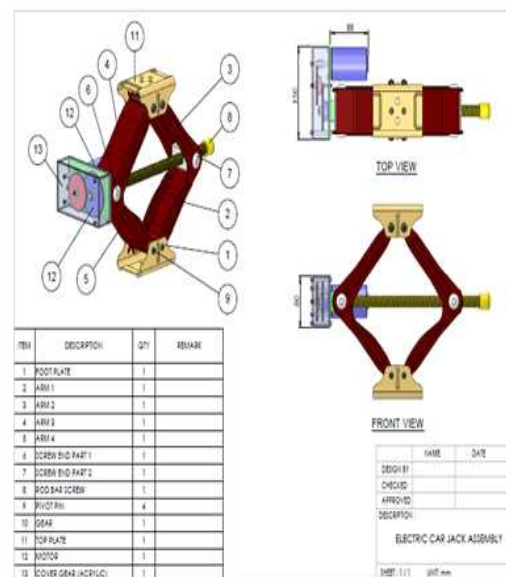
Gambar 3 Gambar kerja Dongkrak Elektrik
