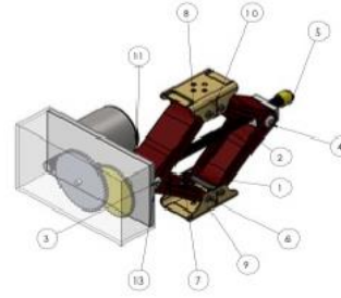
Gambar 2 Sketsa Rancangan Dongkrak
