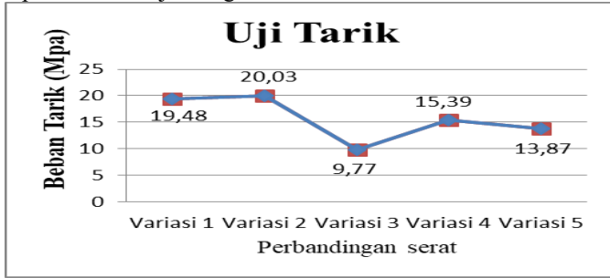
Gambar 7. Grafik Uji Tarik
