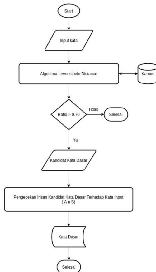
■ Gambar 2 Proses stemming dengan algoritma Levenstein Distance
