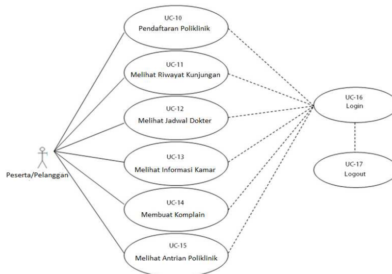
Gambar 4. Usecase Diagram Peserta/Pelanggan
