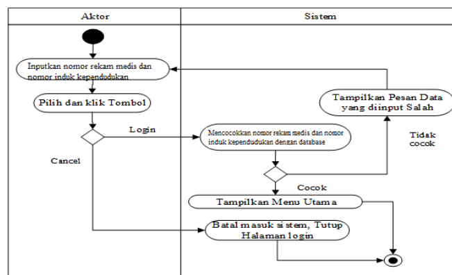
Gambar 5. Activity Diagram Login Peserta/Pelanggan
