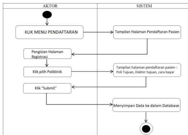
Gambar 6. Activity Diagram Pendaftaran Pasien
