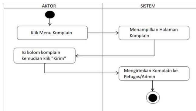
Gambar 10. Activity Diagram Pengaduan Pasien
