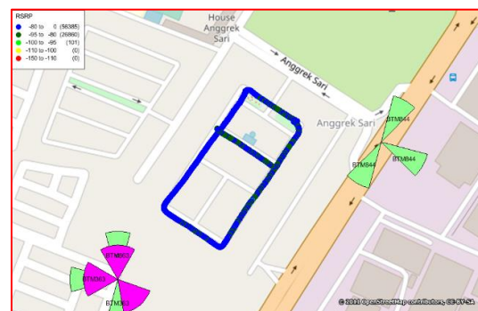
Gambar 7. RSRP setelah optimasi
