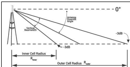
Gambar 4. Batas dalam dan batas luar pancaran antenna
