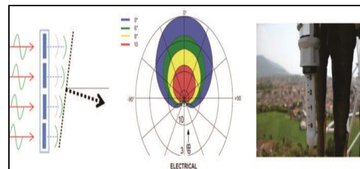
Gambar 2 Perangkat Electrical downtilt dan pengaruhnya pada lobe
