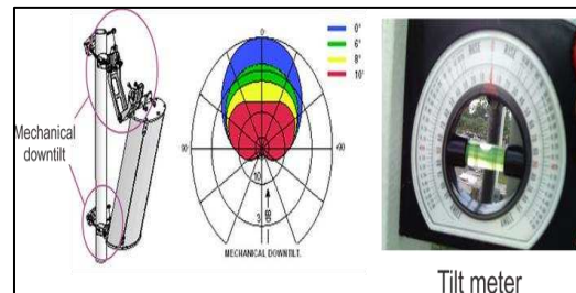
Gambar 1. Perangkat Mechanical downtilt dan pengaruhnya pada lobe
