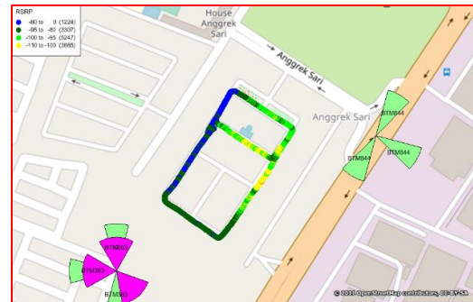
Gambar 6. RSRP sebelum optimasi
