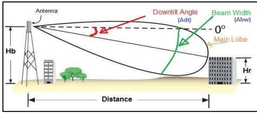
Gambar 3. Jarak dan sudut tilting antenna
