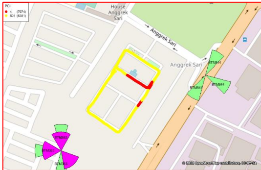
Gambar 8. Cell Identity hasil pengukuran di area keluhan pelanggan
