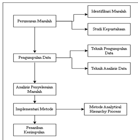
Gambar 1. Tahapan Penelitian
