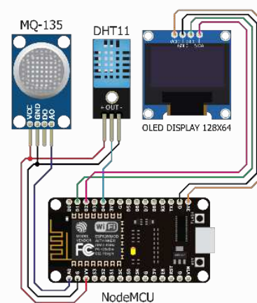
Gambar 1. Skematik Rangkaian Mikrokontroler
