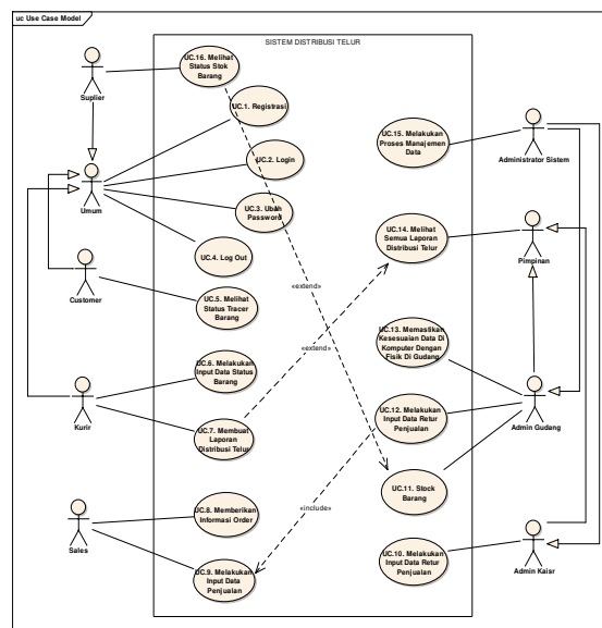
Gambar 3. Sistem Distribusi Telur
