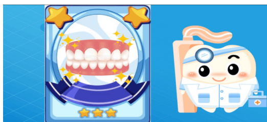
Gambar 14. Interface Gols
