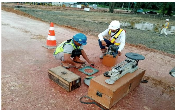
Gambar 14. Pengujian Sandcone
