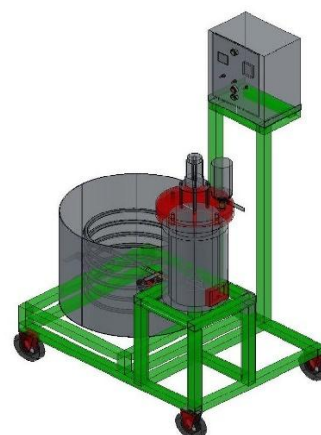
Gambar 2. Ekstraktor Berpengaduk
