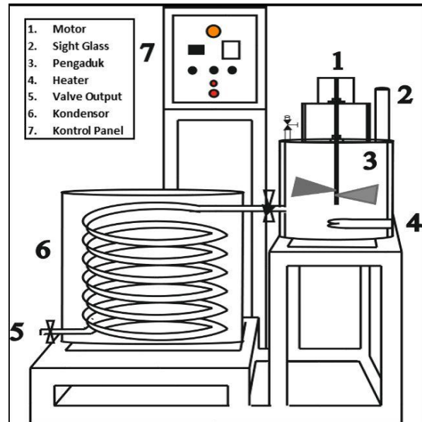
Gambar 1. Ekstraktor Berpengaduk
