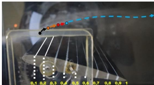
(a) Airfoil tanpa menggunakan Vortex Generator (tampak atas)
