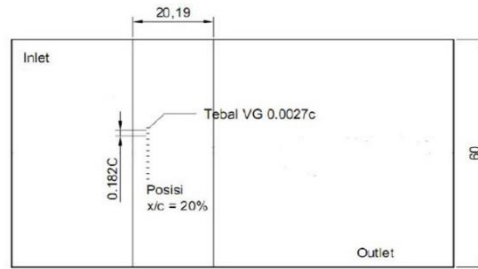
Gambar 2 Posisi peletakan VG pada airfoil
