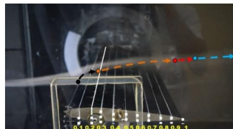
b) Airfoil menggunakan Vortex Generator (tampak atas)
