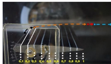
b) Airfoil menggunakan Vortex Generator (tampak atas)
